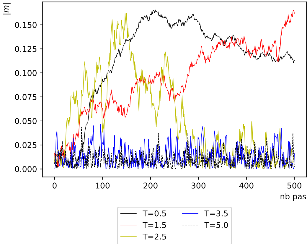
Evolution de l'aimantation sur 500 pas de Monte Carlo, N=128
